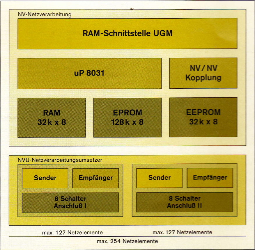
Bild 3 Blockschaltbild der Baugruppe NV 100
