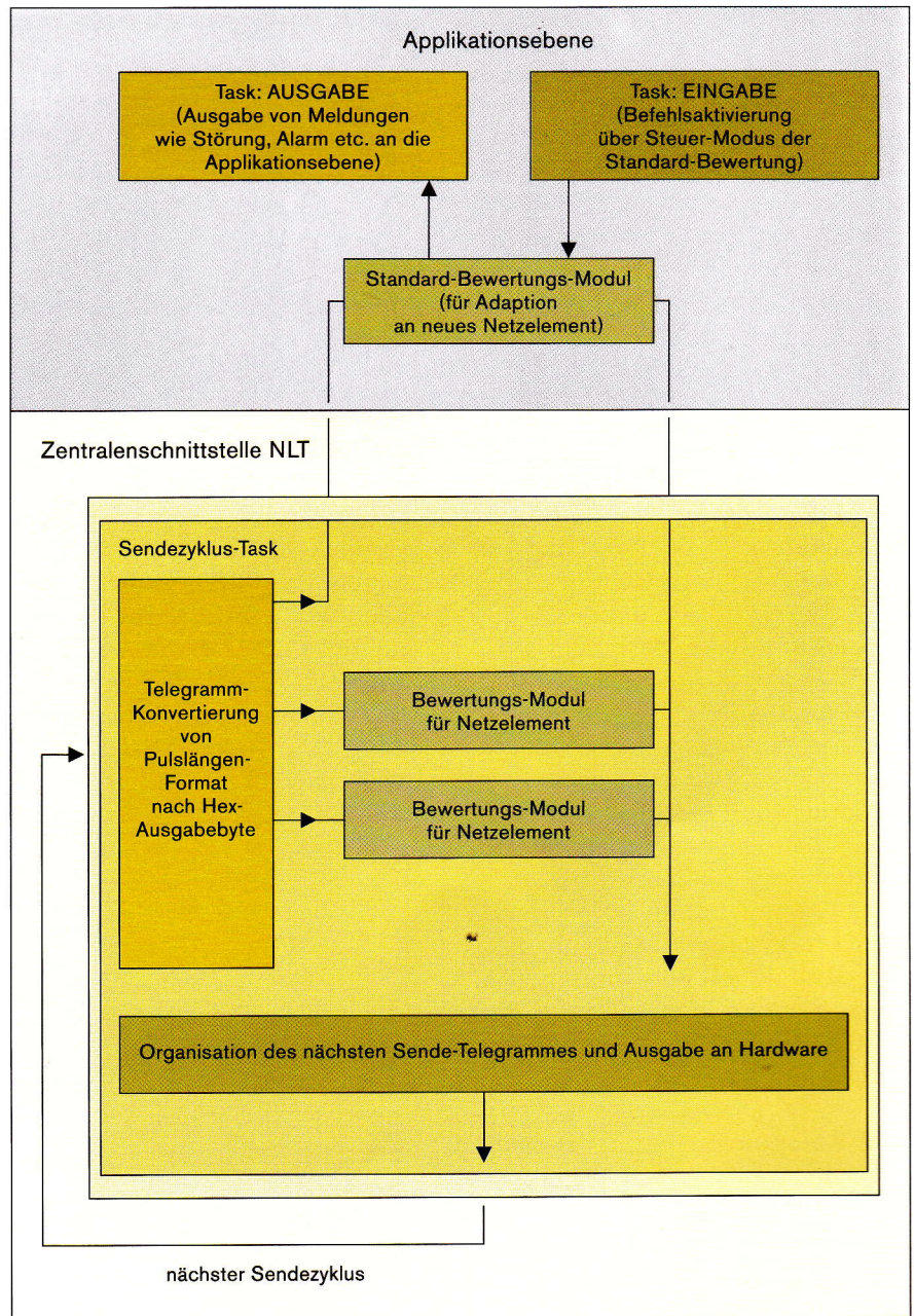
Bild 6 Zentralschnittstelle NLT
