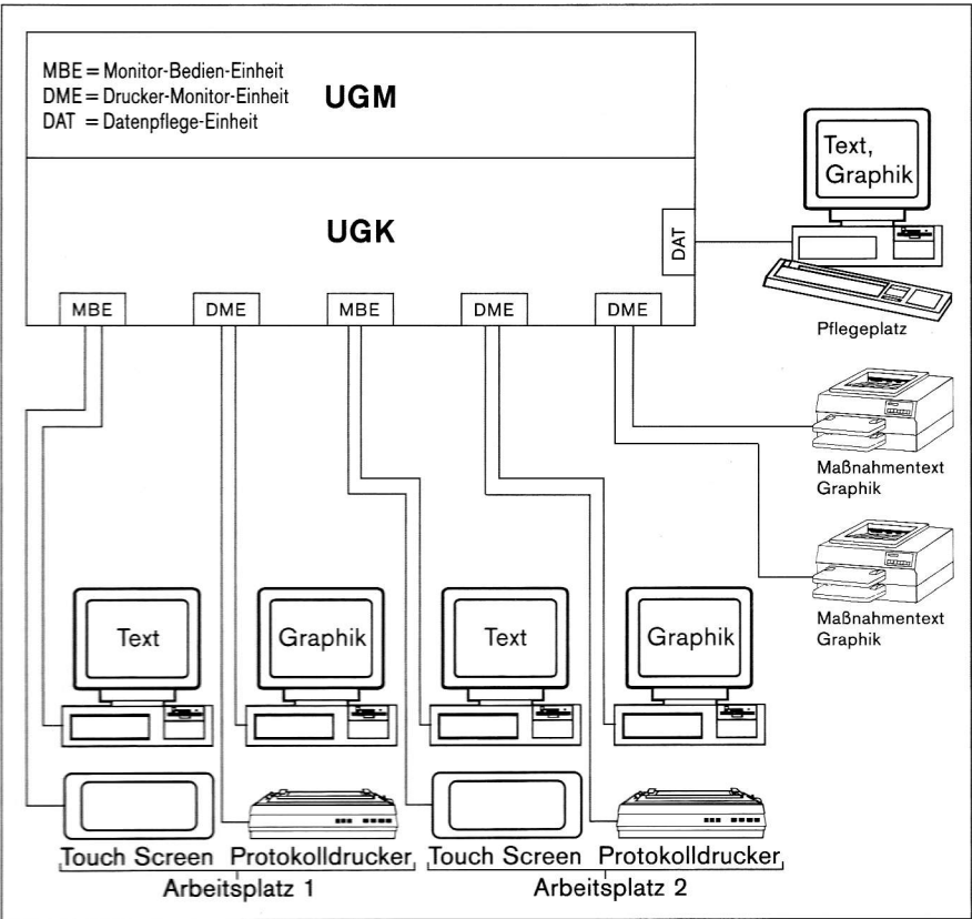
Bild 4 Mehrplatzfähige Bediensysteme mit Touchscreen
