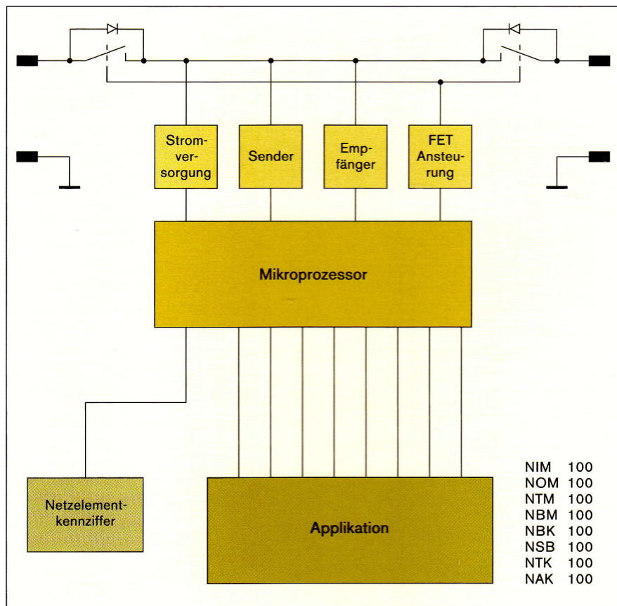
Bild 5 Blockschalbild Netzelement
